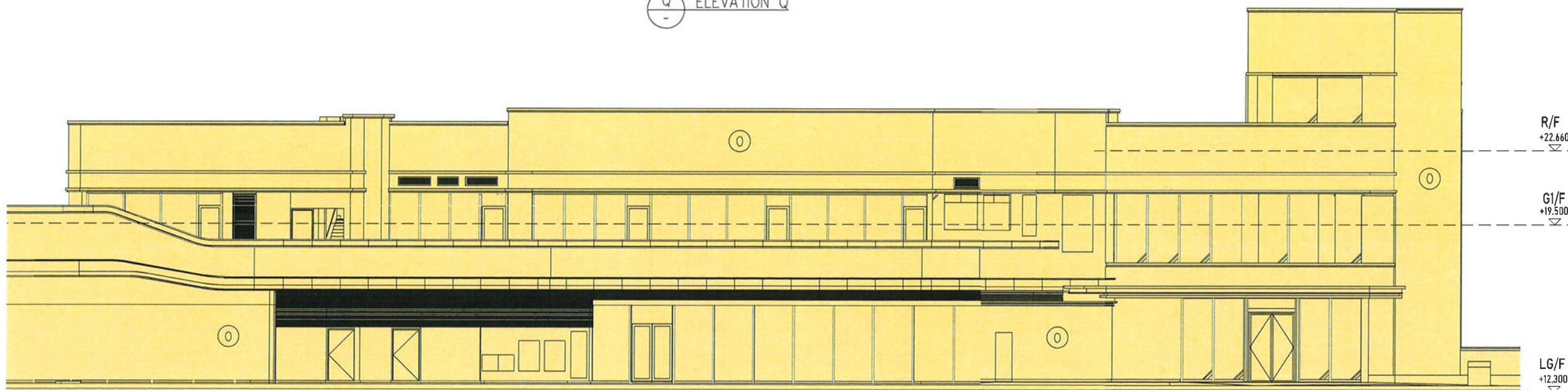
U ELEVATION U
